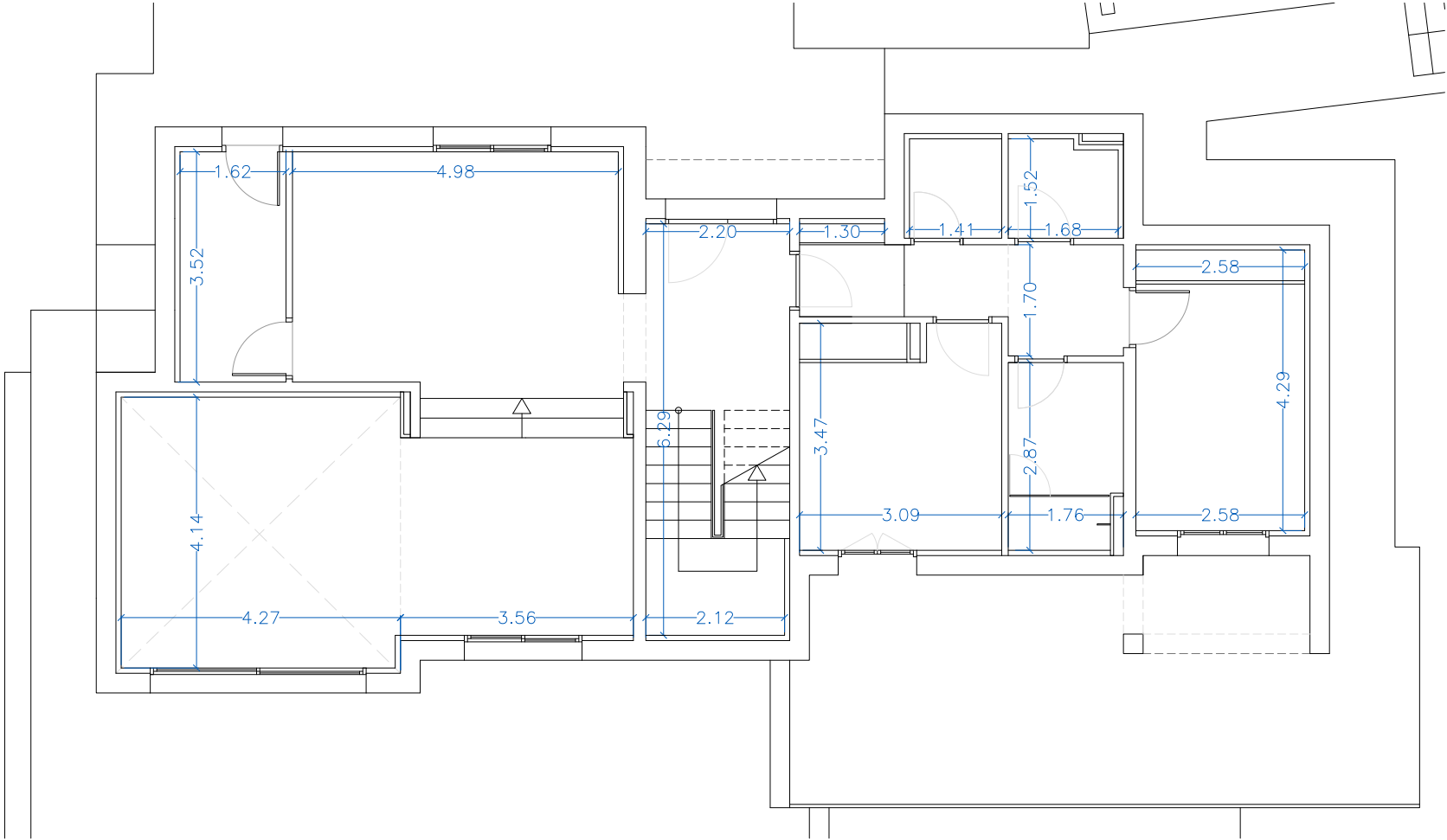
PLANTA BAJA
