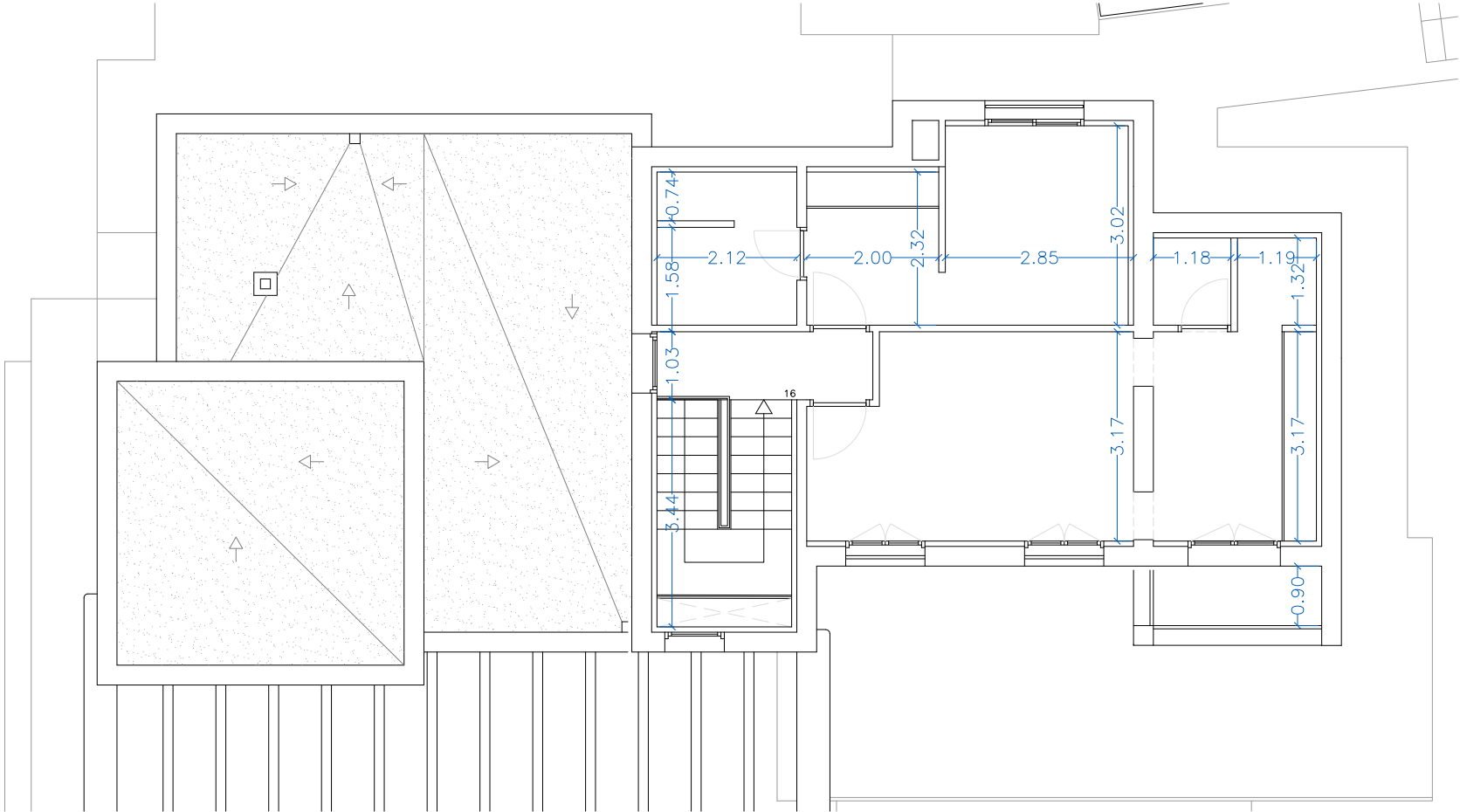
PLANTA PRIMERA
