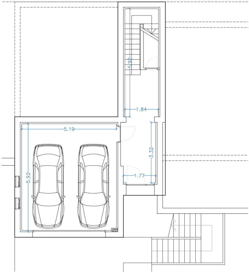
PLANTA SÓTANO
