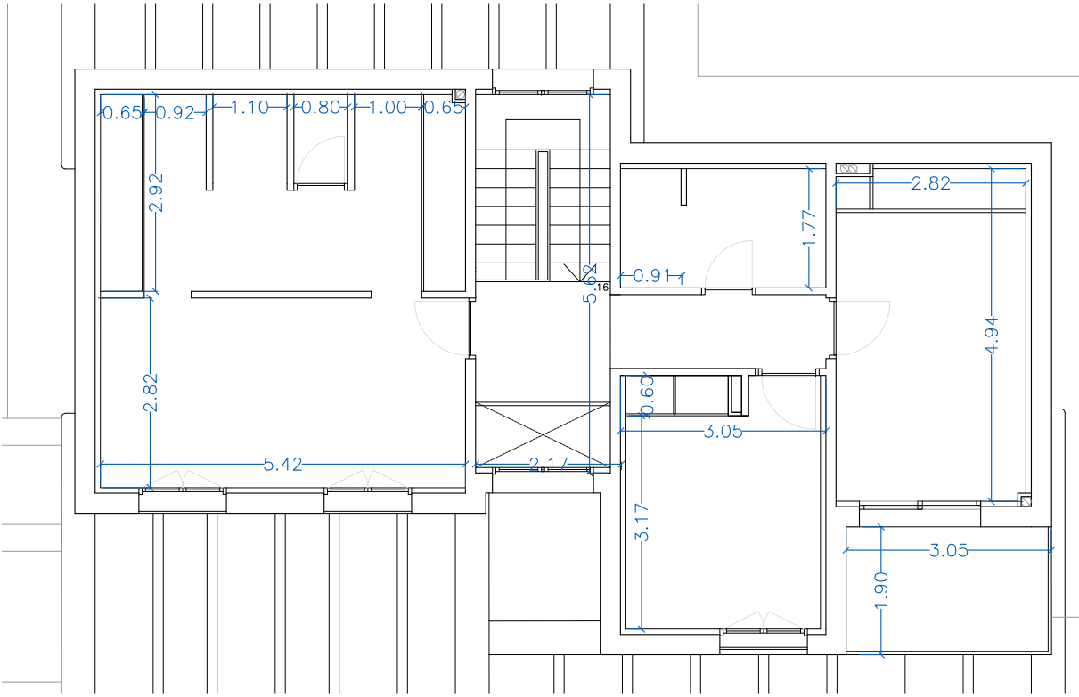
PLANTA PRIMERA
