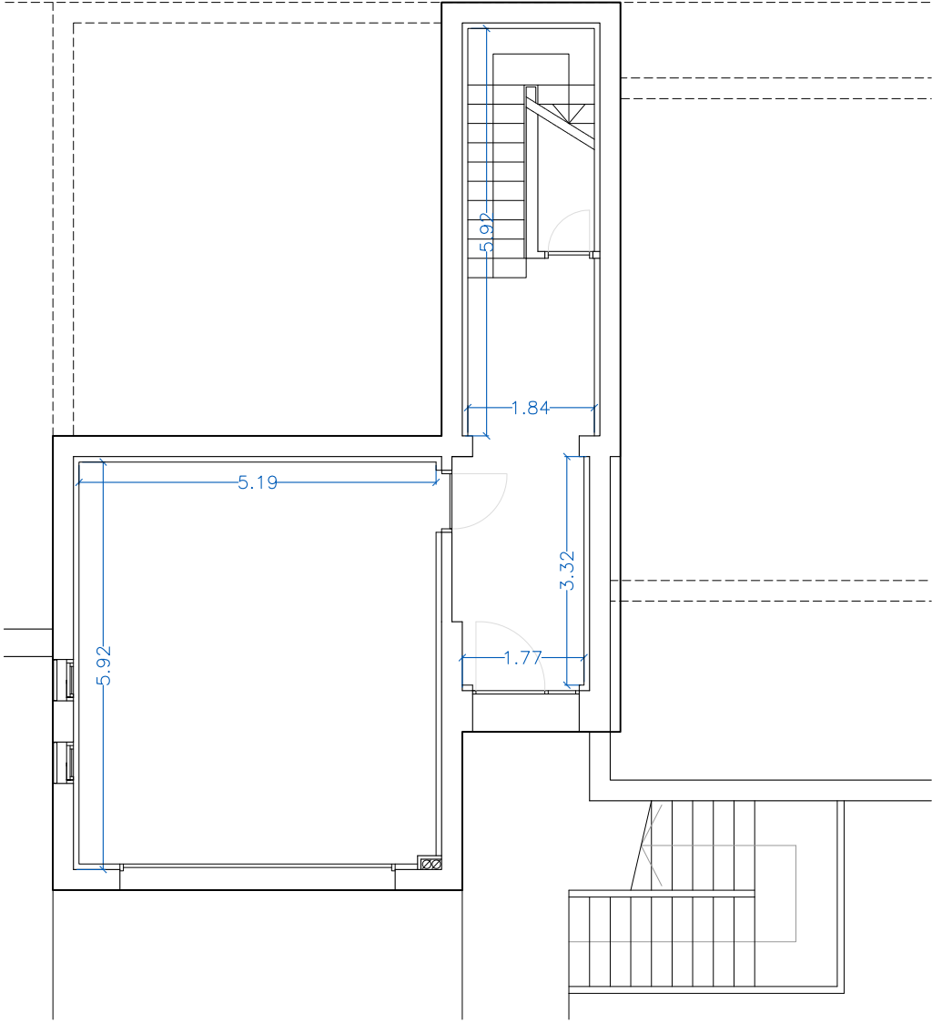
PLANTA SÓTANO
